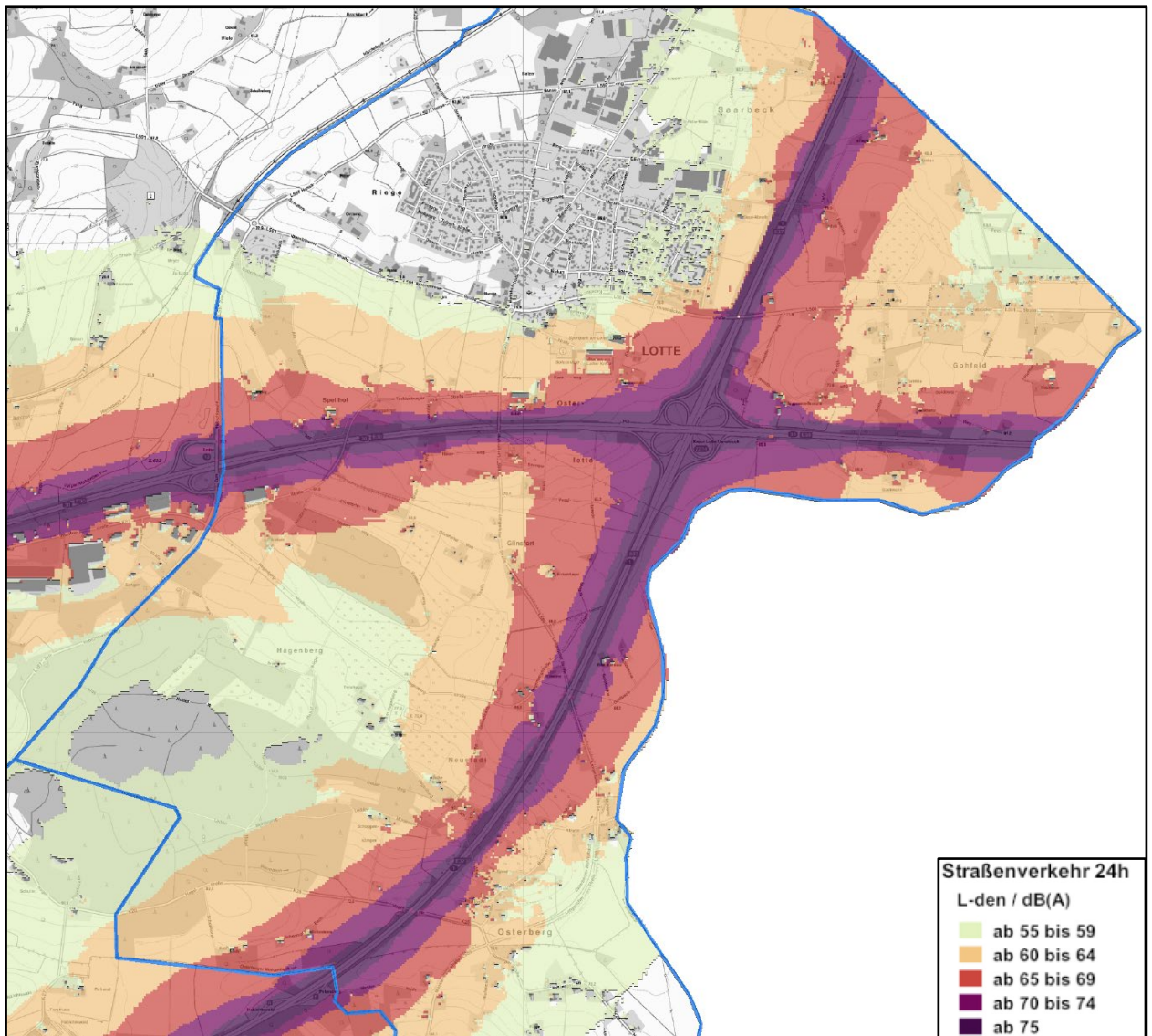
Karte 3: Isophonenkarte Tag L_{den} (24-Stunden) (day, evening, night) für Lotter Kreuz (A 30 und A 1) genordet, ohne Maßstab (Auszug aus Anlage 4)
