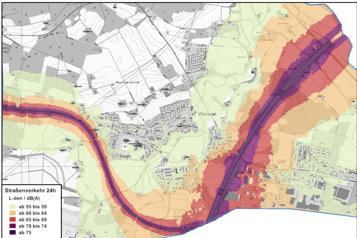
Karte 1: Isophonenkarte Tag L_{den} Wersen (L 595 und A 1), genordet, ohne Maßstab (Auszug aus Anlage 2)
