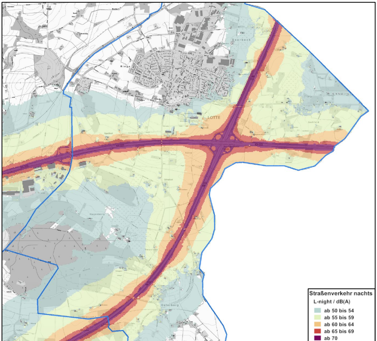
Karte 4: Isophonenkarte Nacht L night (8 Stunden) für Lotter Kreuz (A 30 und A 1) genordet, ohne Maßstab (Auszug aus Anlage 5)
