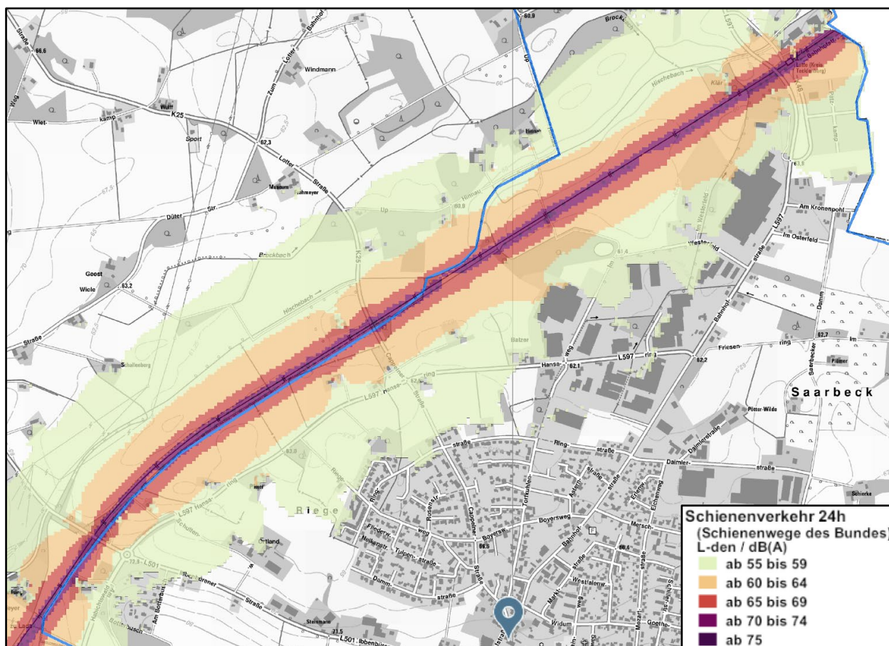
Karte 5: Isophonenkarte Schiene Tag L_{den} (Lotte), genordet, ohne Maßstab (Auszug aus Anlage 6)
