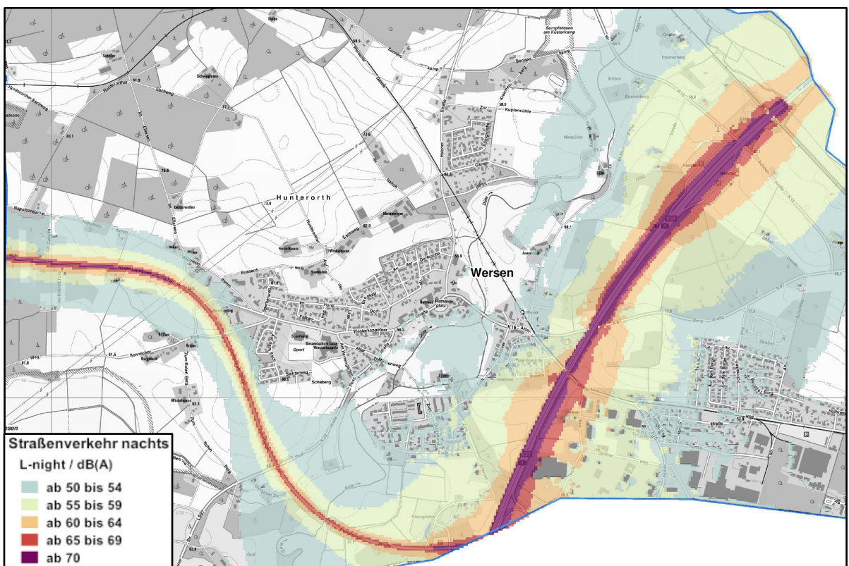
Karte 2: Isophonenkarte Nacht L_{night} Wersen (L 595 und A 1), genordet, ohne Maßstab (Auszug aus Anlage 3)
