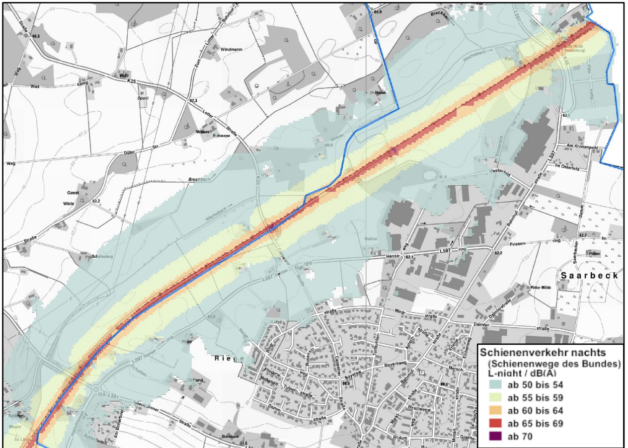
Karte 6: Isophonenkarte Schiene Nacht L_{night} (Lotte), genordnet, ohne Maßstab (Auszug aus Anlage 7)
